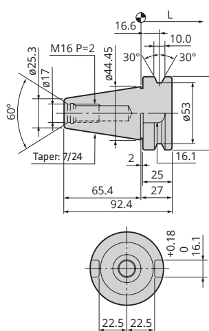
BT40
