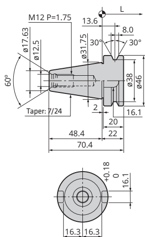
BT30
